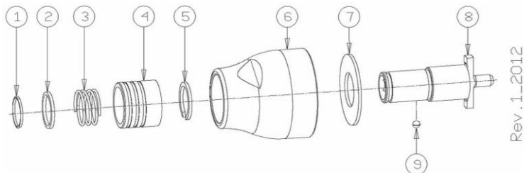
15C - 26C4-5 Gruppo copertina - Cluch case assembly - Groupe carter
