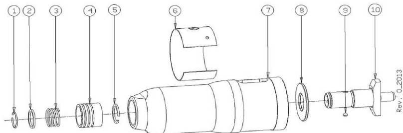
26C8-10-12 Gruppo copertina - Cluch case assembly - Groupe carter
